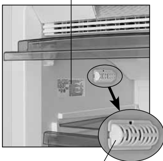
температура сенсоры
