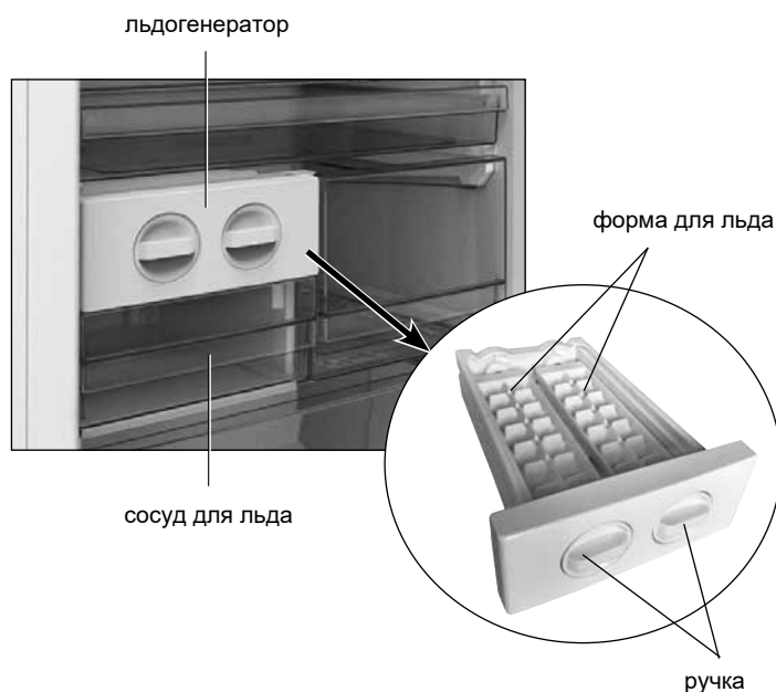
Рисунок 8 – Льдогенератор
