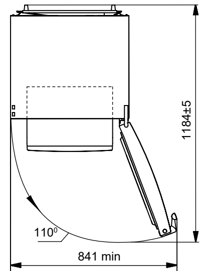
2-сурет – Мұздатқыш (жоғарғы көрініс)
