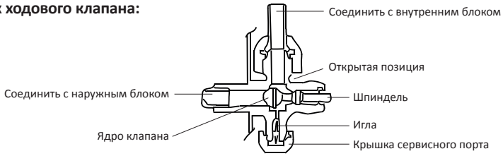
Схема 4-х ходового клапана:
