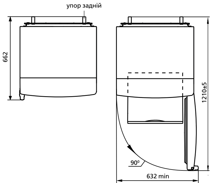
Рисунок 2 – Морозильник (вигляд зверху)
