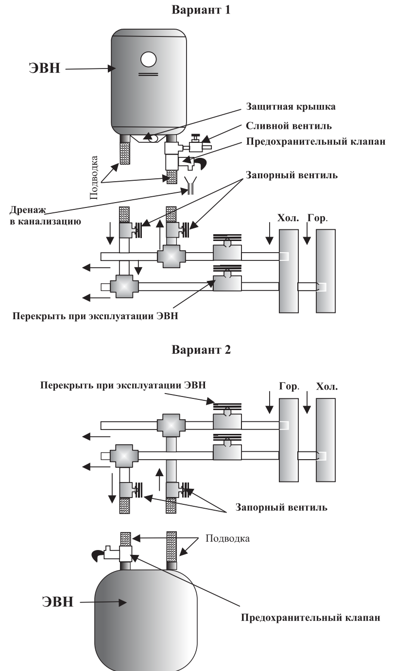
Рис. 1. Схема подключения ЭВН к водопроводу
